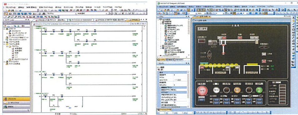
ラダー図
