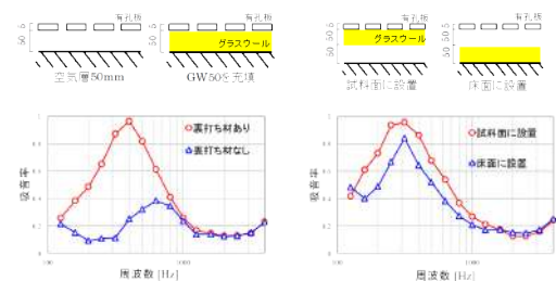
図2 測定結果の例(裏打ち材に関する検討)
