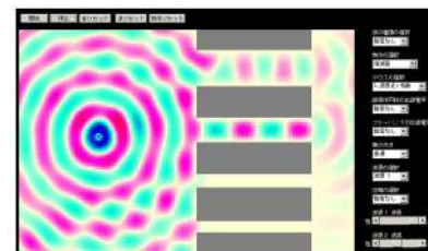
電磁波動画シミュレータの表示画面 (単一周波数の正弦波が幅の異なる複数の導波路に入射した場合の現象をシミュレーションしたもの。赤い部分が正、青い部分が負の値を表す。)
