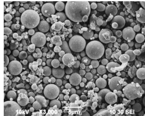
改質フライアッシュの 電子顕微鏡写真
