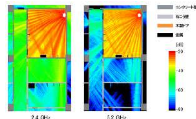
無線LAN電磁波の屋内伝搬シミュレーション (周波数によって干渉縞の間隔や壁面での透過率が異なる様子がわかる。)
